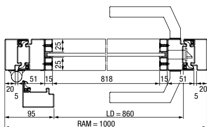
1-szárnyú acél Loftajtó vízszintes metszete
