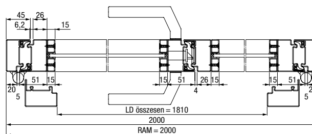
2-szárnyú acél Loftajtó vízszintes metszete
