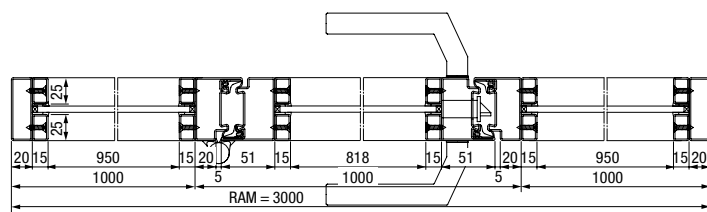
Oldalelemekkel és felülvilágítóval ellátott 1-szárnyú acél Loftajtó vízszintes metszete
